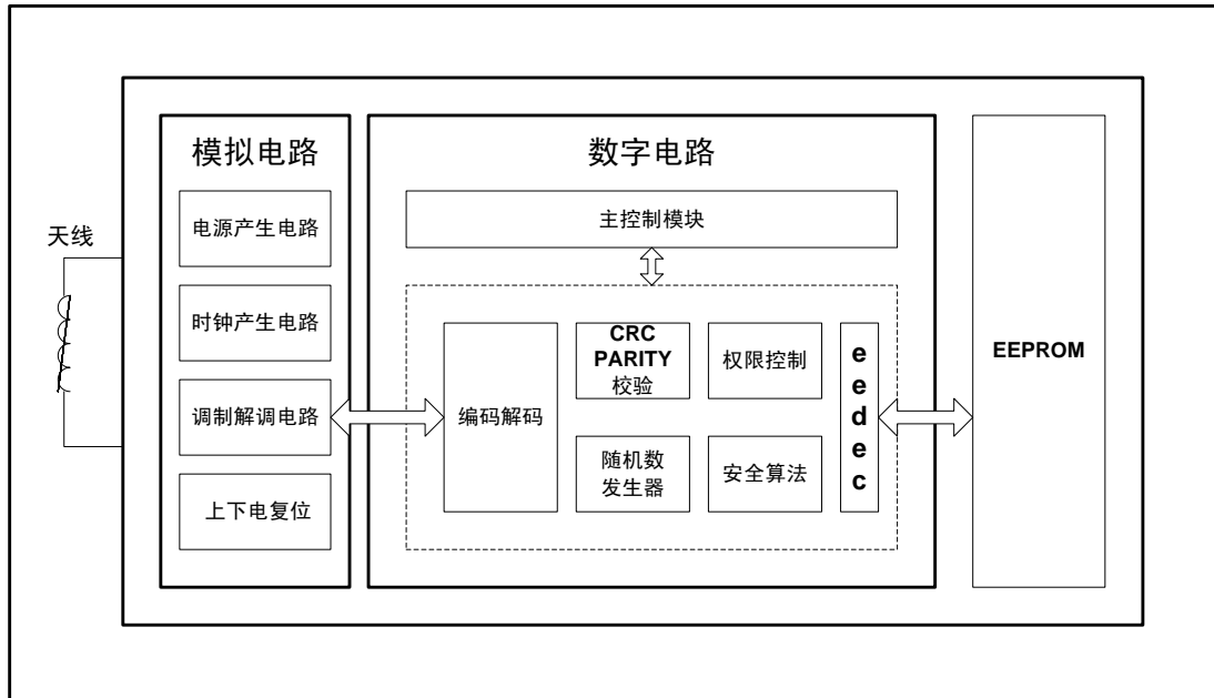
图 1-1 FM11S08 功能框图
