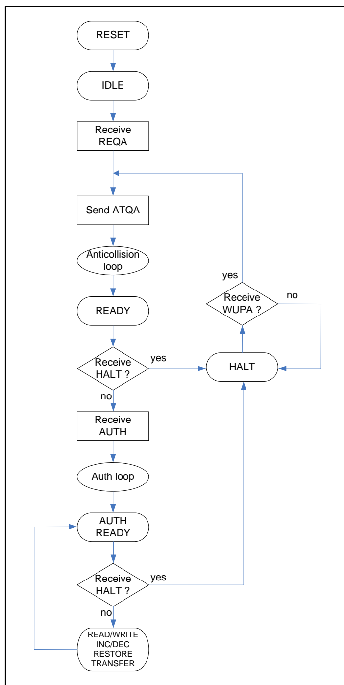
图 2-1 FM11S08 芯片 workflow
